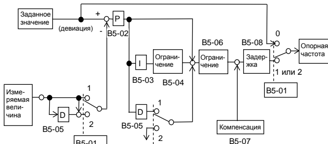
Схема ПИД-регулирования
